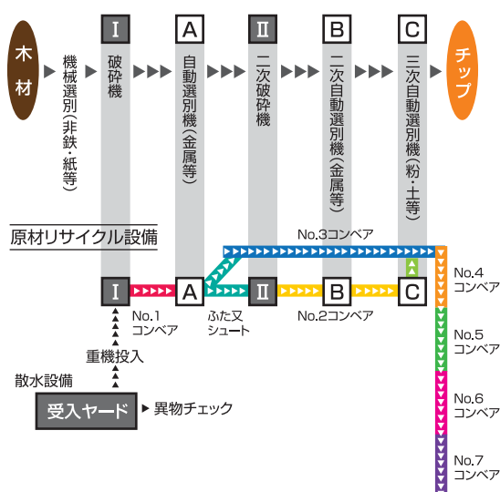
木材再生システム(フルオートメーション)
